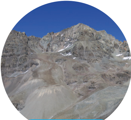
Glaciar rocoso
