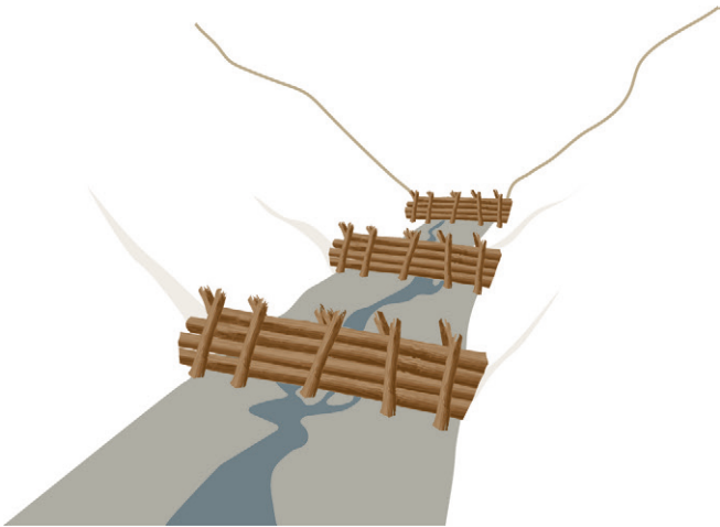
Barreras de control aluvional: Son estructuras de protección contra aluviones de diversos diseños y materiales, como hormigón, madera-piedra o gaviones de bolones. Su función es amortiguar y dividir un flujo de detritos y, a la vez, retener los bloques de mayor tamaño, dejando pasar la fracción líquida y sedimentos finos solamente. Comúnmente se instalan de forma escalonada una serie de estas estructuras a lo largo de un cauce.
